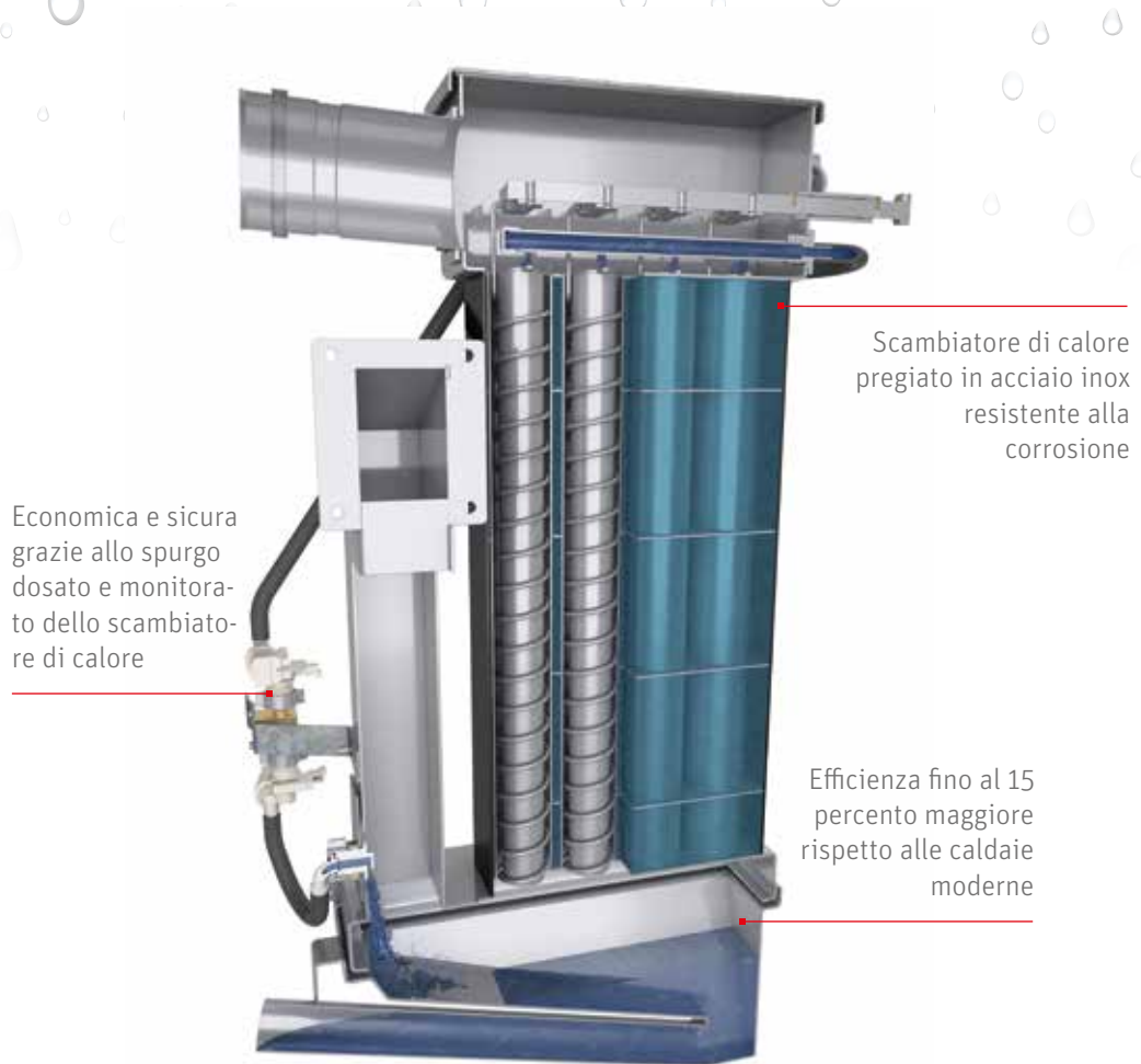
01. Sezione dello scambiatore di calore a condensazione
