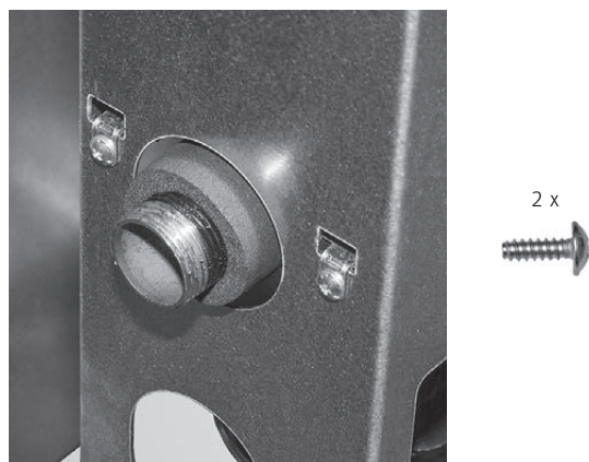
Fig. 57 Piegare le linguette verso il basso e avvitare saldamente – vista dal retro
