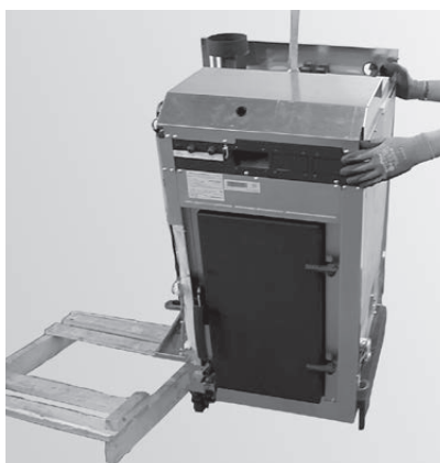
Fig. 15 Sollevamento della caldaia dal pallet
