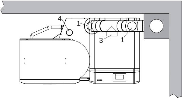
Fig. 115 Raccordo gas combusto verso l'alto – vista dall'alto, (schizzo senza isolamento del tubo dei gas combusto)
