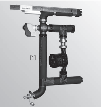
Fig. 52 Gruppo idraulico
