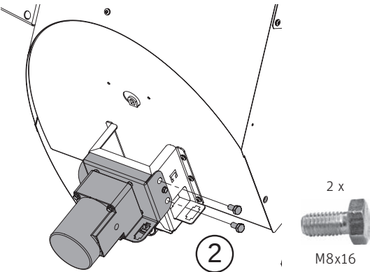
Fig. 42 Avvitare il motore della coclea
