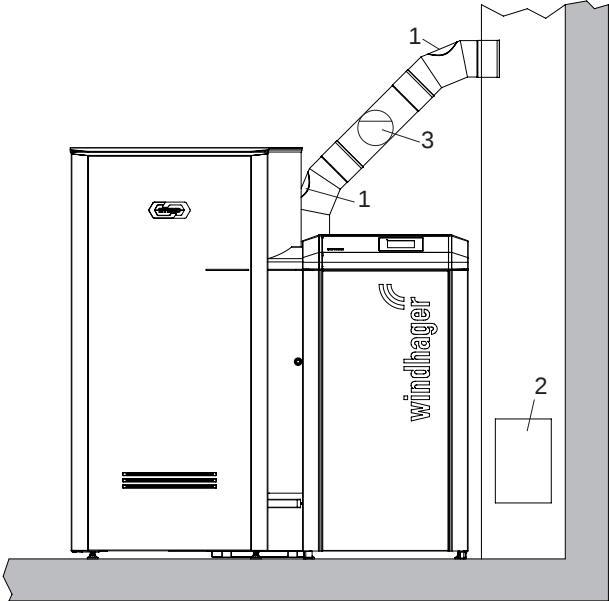
Fig. 113 Raccordo gas combusto verso l'alto – vista da davanti, (schizzo senza isolamento del tubo dei gas combusto)
