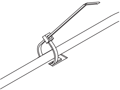
Fig. 129 Fissare i cavi con una fascetta per cavi come scarico della trazione
