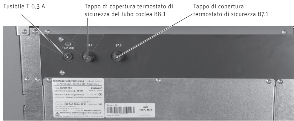
Fig. 117 Quadro di comando BioWIN 2 Hybrid
