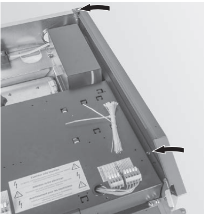
Fig. 99 Infilare la parte superiore del rivestimento e avvitare
