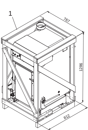
Fig.2 Caldaia
