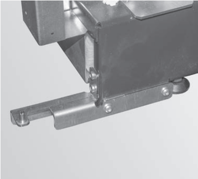
Fig. 95 Avvitare la cerniera della porta in basso
