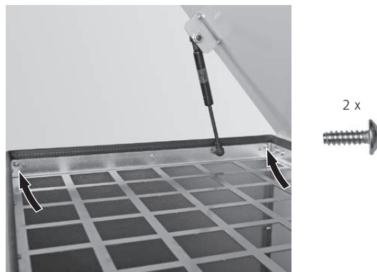
Fig. 89 Avvitare saldamente la parete laterale a sinistra in alto all'interno del serbatoio settimanale con 2 viti
