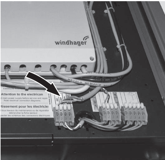
Fig. 125 Collegamento Modbus su BioWIN 2 Hybrid
