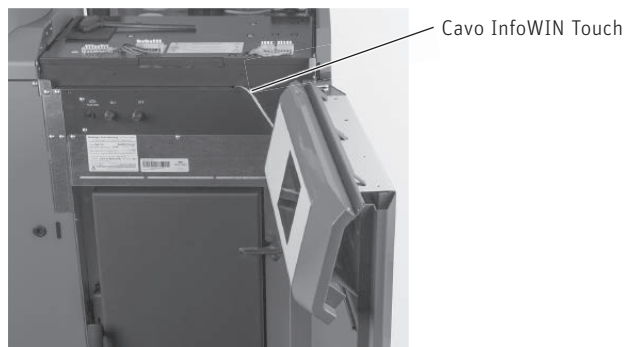
Fig. 121 Agganciare il pannello di comando alla porta (posizione di assistenza), aprire il coperchio
