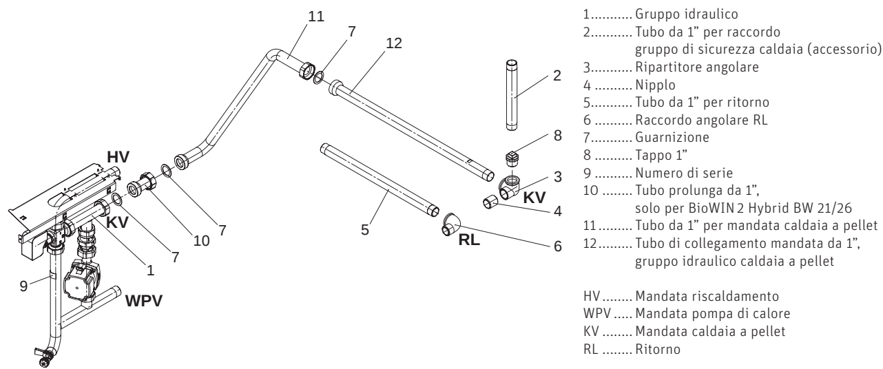
Fig. 51 Gruppo idraulico
