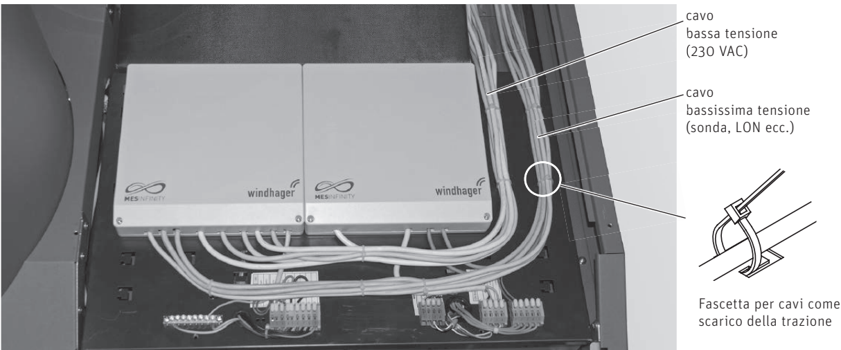
Fig. 133 Cablaggio BioWIN2 Hybrid con regolazione nel quadro di comando della caldaia
