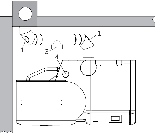
Fig. 114 Raccordo gas combusto verso il retro – vista dall'alto, (schizzo senza isolamento del tubo dei gas combusto)
