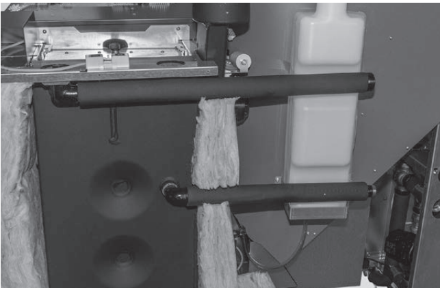
Fig. 63 Impermeabilizzare il tubo di collegamento mandata e il tubo di ritorno
