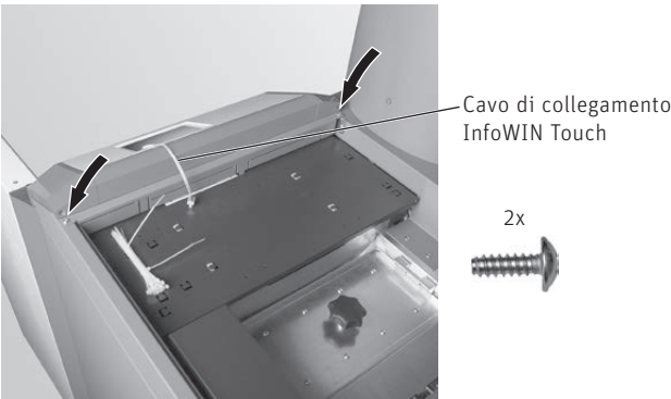
Fig. 102 Infilare il cavo di collegamento, agganciare il pannello di comando e avvitarlo
