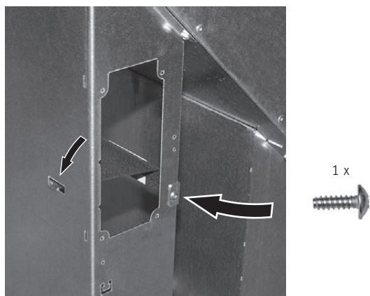
Fig. 56 Inserire la linguetta nella cavità e fissare sul davanti con una vite autofilettante – vista da davanti
