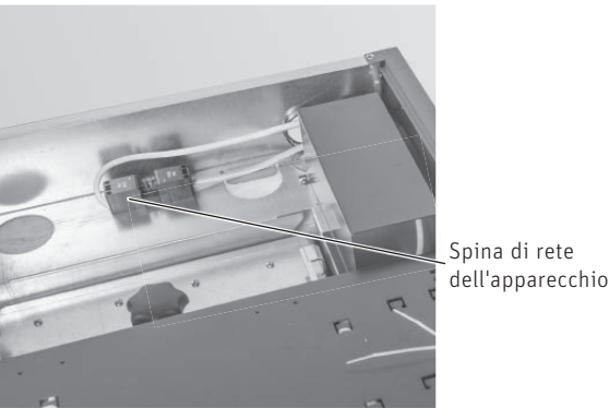
Fig. 136 Inserire risp. collegare la spina di rete
