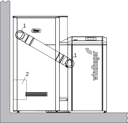
Fig. 112 Raccordo gas combusto verso il retro – vista da davanti, (schizzo senza isolamento del tubo dei gas combusto)
