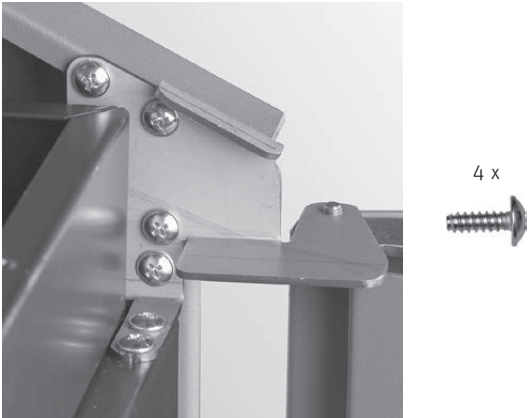
Fig. 101 Serrare la cerniera della porta in alto, avvitare la parete laterale con 4 viti autofilettanti
