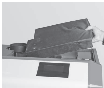
Fig. 119 Rimuovere l'isolamento
