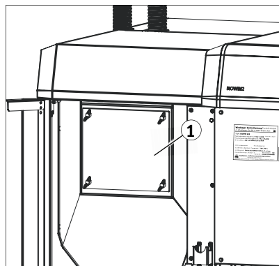
Fig. 63 Rimuovere i dadi ad alette e togliere il coperchio di revisione
