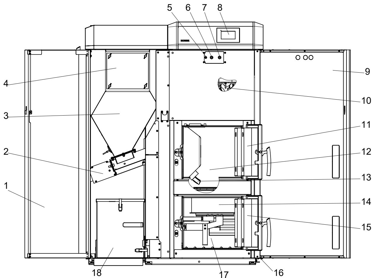
Fig.10 BioWIN2 DELUXE con una porta di contenimento e senza sportelli camera di combustione
