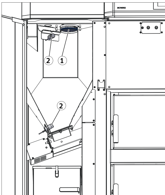
Fig. 64 Rimuovere la polvere dal filtro grossolano, rimuovere la polvere dall'interruttore superiore e inferiore del livello di riempimento
