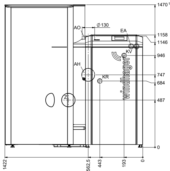
Vista posteriore:
