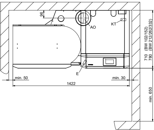
Vista in pianta, Distanze minime: (tubo dei gas combusti verso l'alto*)
